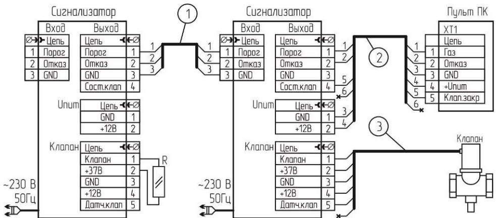
R – имитатор клапана (резистор типа С2-33-0,125-100 Ом-20% из комплекта поставки) 1 – Кабель типа КСПВ 4х0,52 (УТР-2) 2 – Кабель типа КСПВ 6х0,52 3 – Кабель клапана (см. рисунки В.3, В.4)
