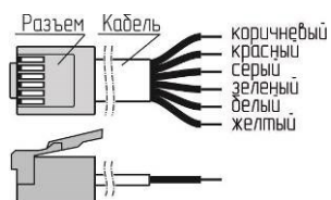
Вилка на кабель TP6P6C (цветовая маркировка проводов)
