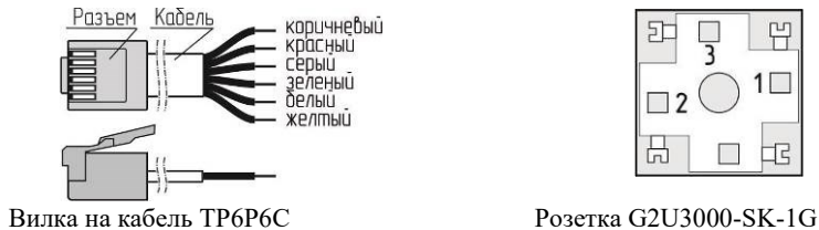
Рисунок В.3 – Обозначение контактов разъемов
