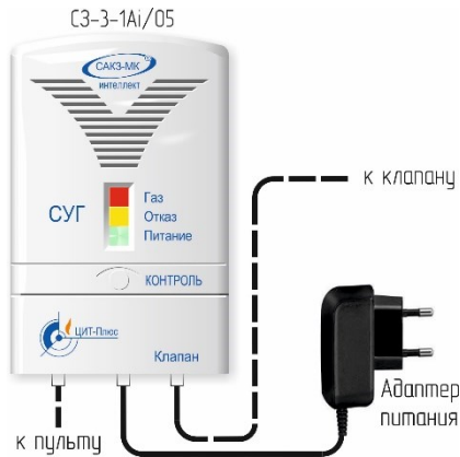
Рисунок Б.1 – Типовая схема включения сигнализатора
