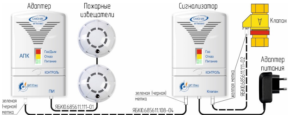
Рисунок Б.2 – Типовая схема подключения пожарных извещателей
