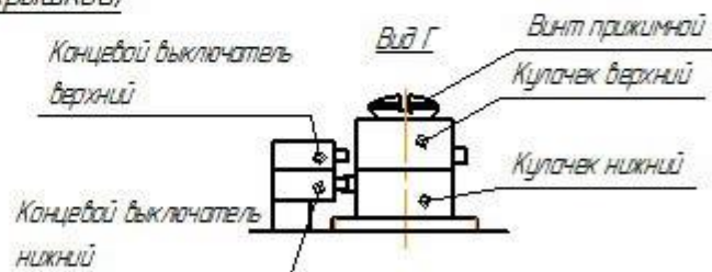
д) Регулируемые кулачки и концевые выключатели
