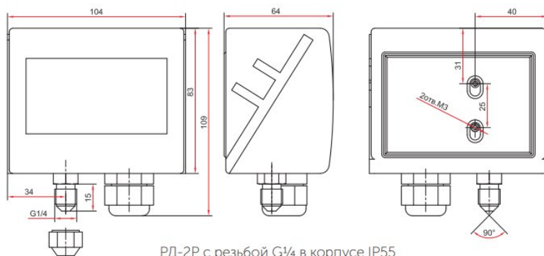
РД-2Р с резьбой G1/4 в корпусе IP55
