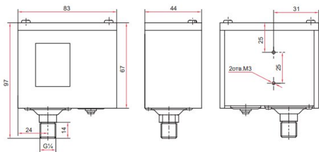
Реле давления РД-2Р-0,6 / 0,8 / 1,6 МПа модель 35 с резьбой G1/4
