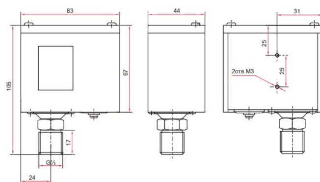
Реле давления РД-2Р-0,8 МПа модель 35 с резьбой G1/2
